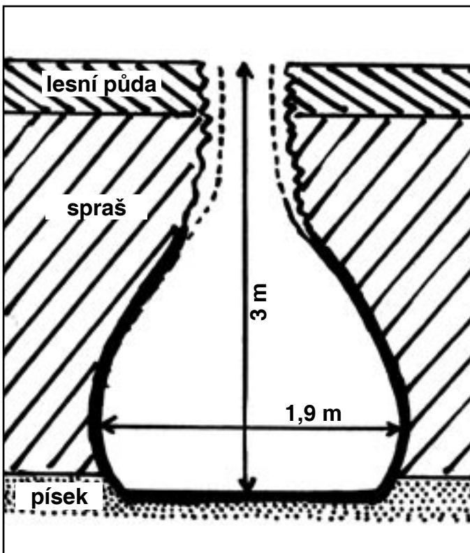
Schema obilní jámy z lesnického Hájku. Předpokládaný tvar sesutého ústí obilnice je naznačen přerušovanou čarou.
